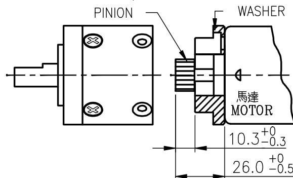
馬達裝卸方法 / MOTOR INSTALLATION
