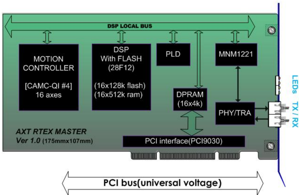
그림 2. PCI-R1604 블록도
