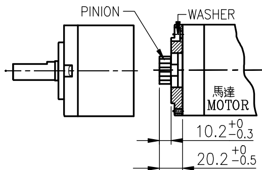
馬達裝卸方法 / MOTOR INSTALLATION
