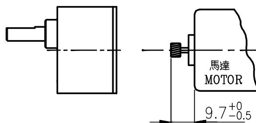
馬達裝卸方法 / MOTOR INSTALLATION
