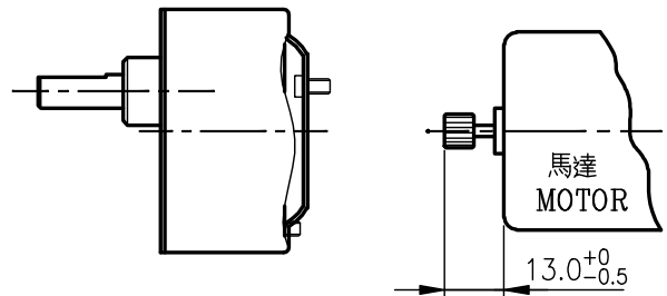
馬達裝卸方法 / MOTOR INSTALLATION
